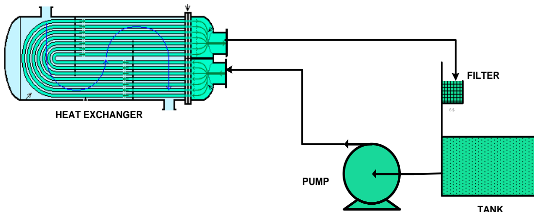
Sơ đồ lắp đặt thiết bị tuần hoàn
